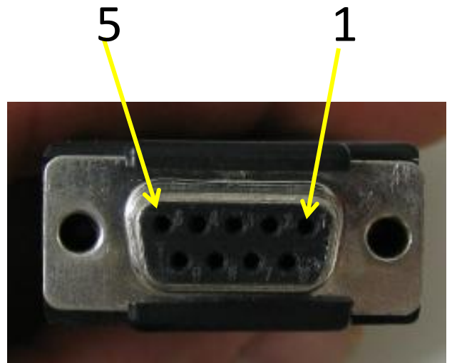
Stecker RS232
