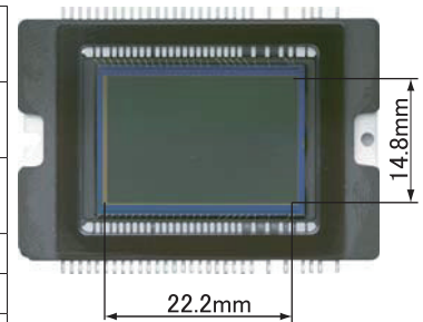
Fig. 001 CMOS sensor
