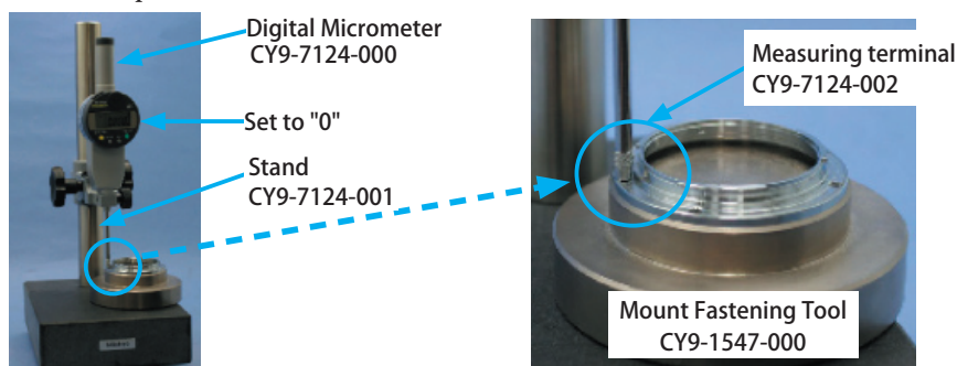
Fig. 003 Set up
