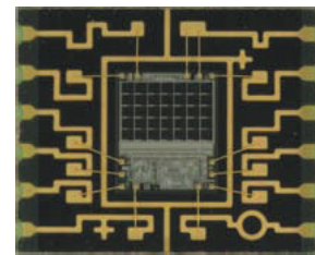
Fig. 016 Metering sensor
