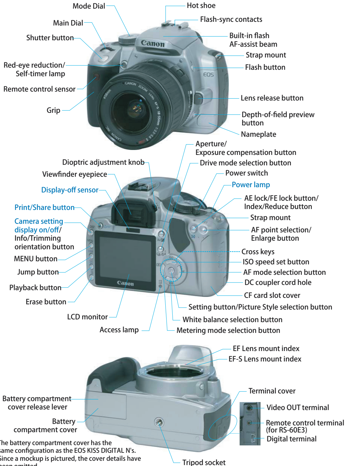
Fig. 024 Nomenclature
