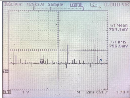
Pin 3 Kontrast gegen GND
