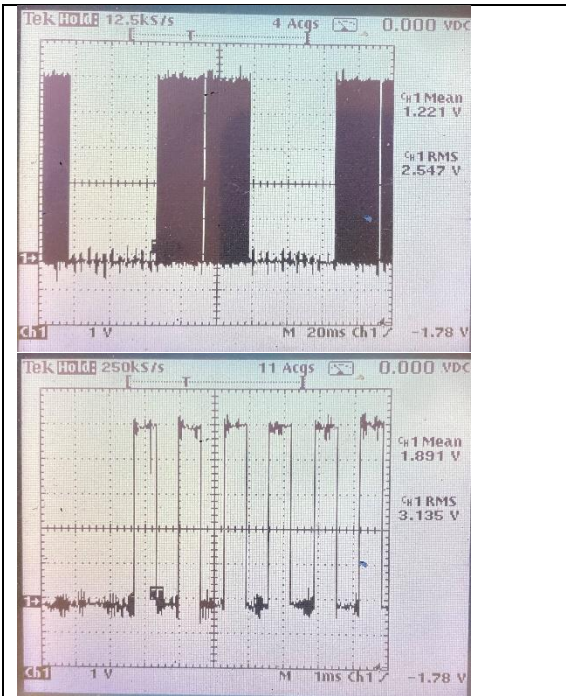
Pin 5 R/W gegen GND
