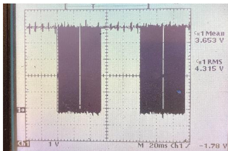
Pin 3 Kontrast gegen GND
