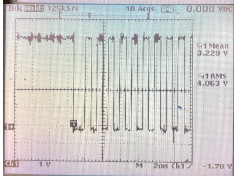
Pin 4 RS gegen GND
