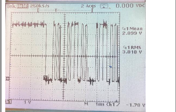
Pin 11 Datenleitung 4 gegen GND
