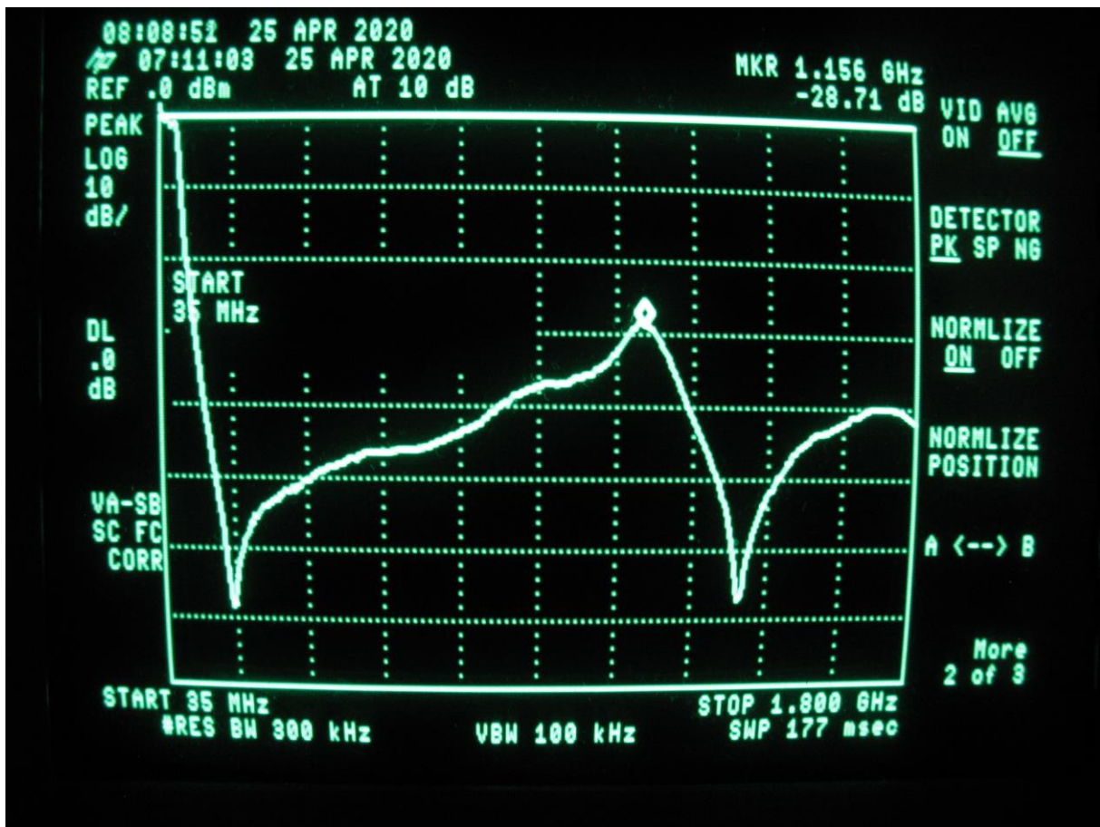
HP8591E Peak Detect / Normalize (Pegel ADF4351 von Kurve subtrahiert)
