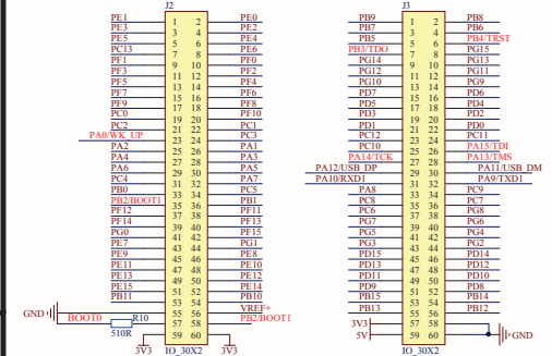
extend I/O
