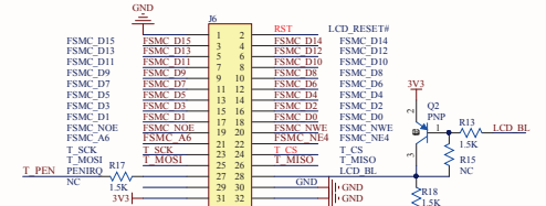
TFT I/F
