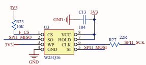
FLASH-W25Q16
